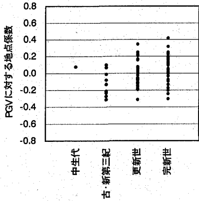
(b) 最大速度
