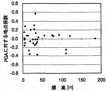
(a) 最大加速度
