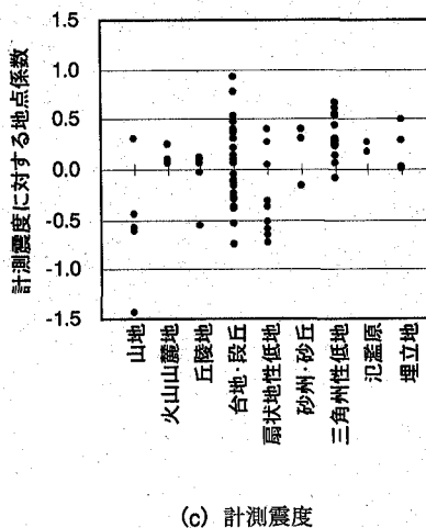
図-3 地点係数と地形分類の関係
