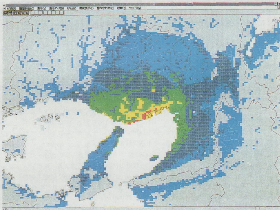
図-12 国土庁の地震被害早期評価システム(EES)で推定した兵庫県南部地震の震度分布
