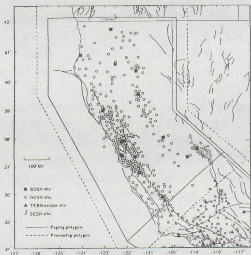
図-14 REDIシステムの地震観測点 36)
