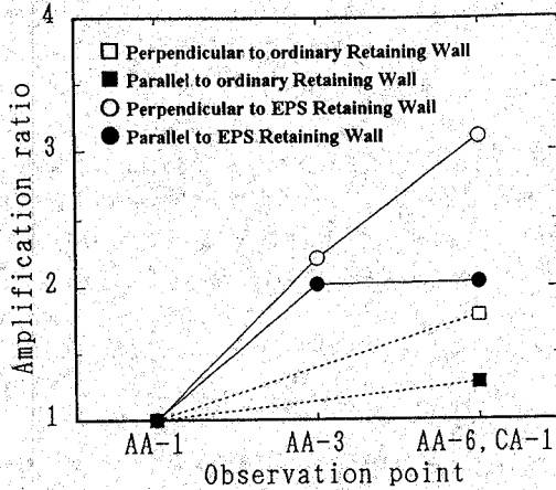
図-8 EPS擁壁と通常擁壁の近傍地盤における最大加速度の増幅傾向の比較(63地震の平均)
