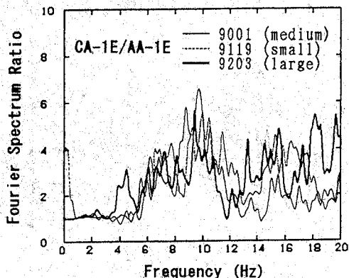
図-11 3地震で観測されたAA-1Eに対するCA-6Eのフーリエ振幅比
