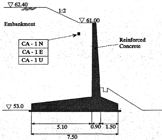
図-3 通常擁壁の断面と地震計配置
