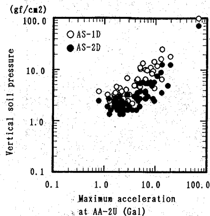
図-13 上下成分の最大加速度とEPS擁壁底面の最大土圧
