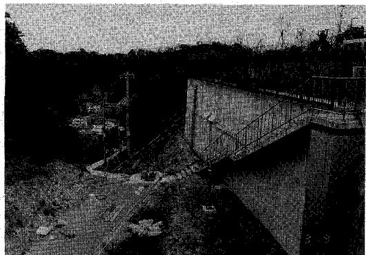
写真-1 EPS盛土の鉄筋コンクリート擁壁外観
