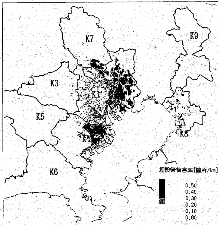
図-13 想定地震による各メッシュの埋設管被害率
