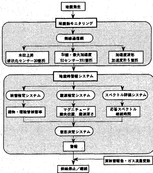
図-3 SIGNALのシステム構成とフロー
