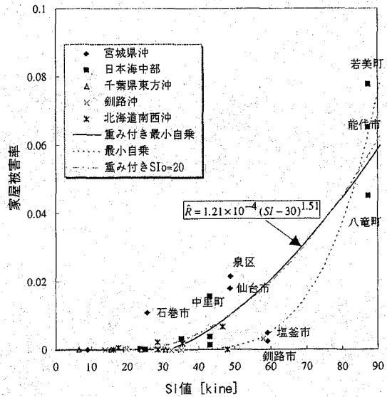
図-4 SI値と家屋被害率の関係
