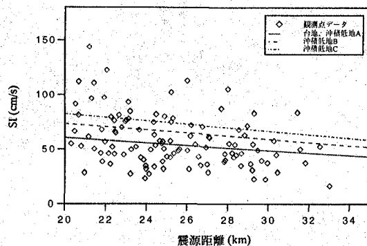
図-12 想定地震におけるSI値と震源距離の関係
