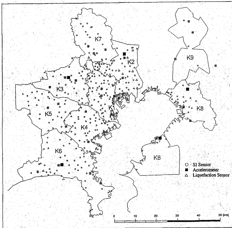
図-2 都市ガス供給網の中圧ブロックとモニタリング用地震センサー
