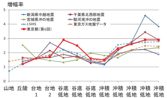
図 9 広域地盤データと地震記録から推定される地盤増幅率と東京都地盤増幅率（第 6 回）の比較
