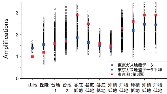
図6 東京都地盤増幅率(第6回)と東京ガス地盤データより推定される増幅率の比較
