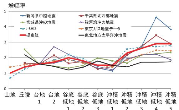
図 13 東北地方太平洋沖地震の観測値より推定された地盤増幅率と本研究の検討結果の比較
