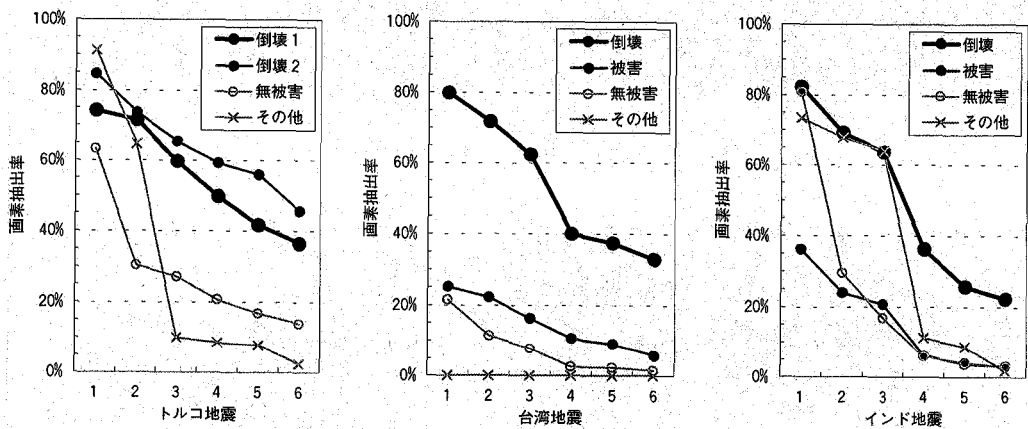
図-12 地震災害画像ごとに設定した閾値を用いた場合の画素抽出率の変化。1=色相，2=1+彩度，3=2+明度，4=3+エッジ強度，5=4+エッジ強度の分散，6=5+エッジ方向の最頻度。
