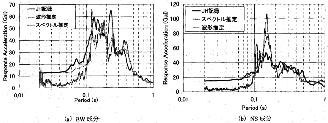
図-17 JH山武成東ICにおける観測地震動と推定地震動の加速度応答スペクトル(5%減衰)の比較
