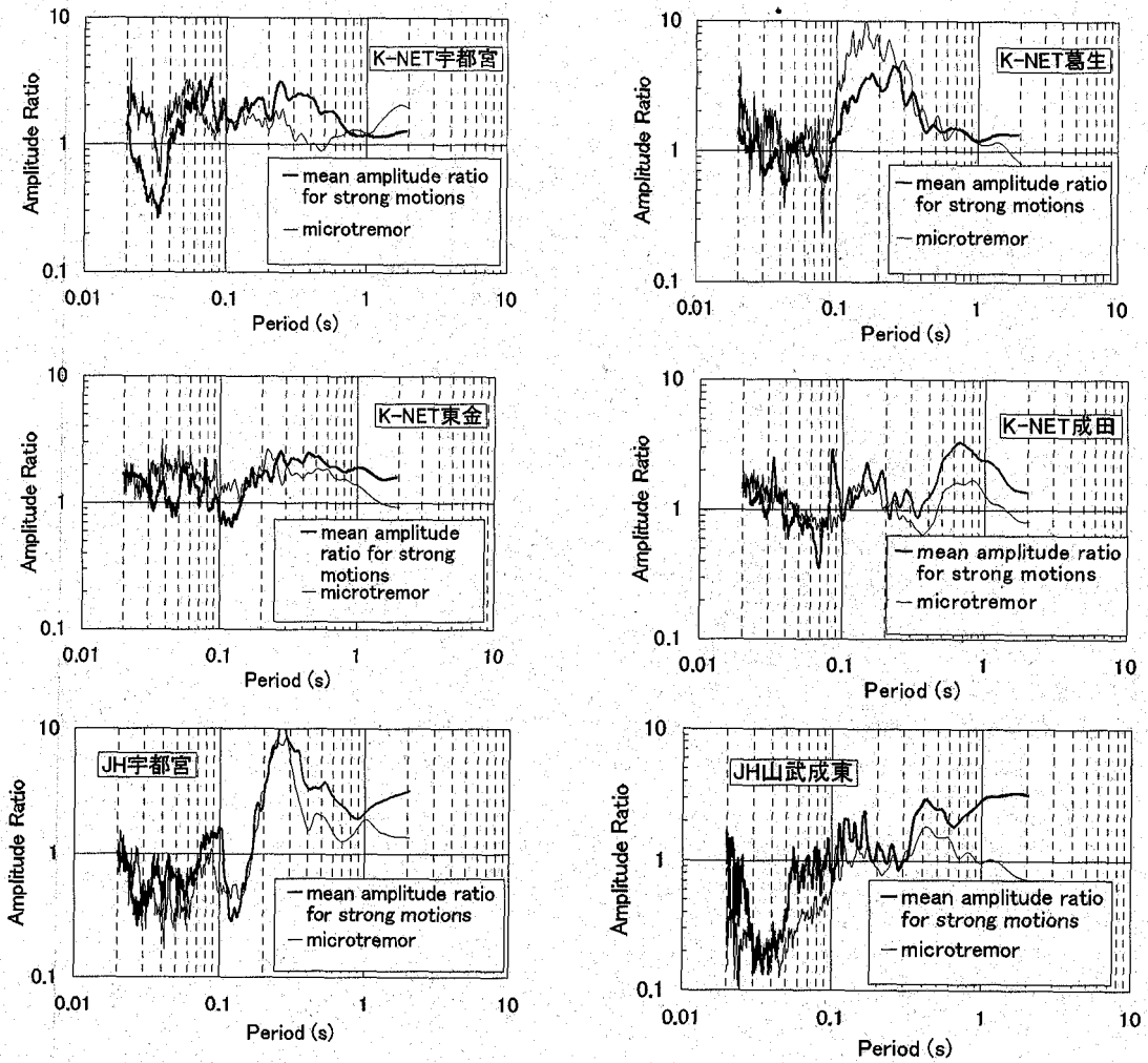
図-6 常時微動と地震動のH/Vスペクトル比の比較
