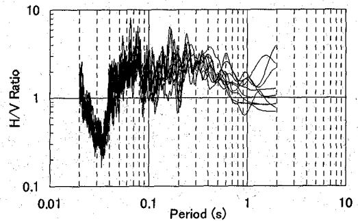
図-5 K-NET 宇都宮における地震動 H/V スペクトル比
