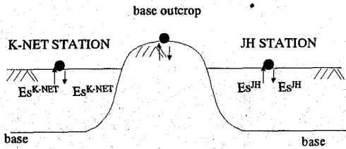
図-8 共通基盤を有する2地点の地盤モデル
