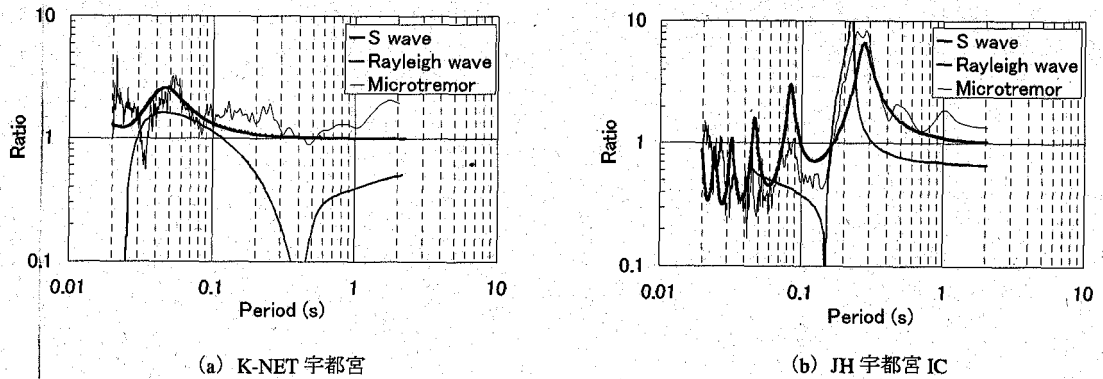
図-7 常時微動のH/Vスペクトル比とRayleigh波基本モードH/Vスペクトル比、S波伝達関数の比較
