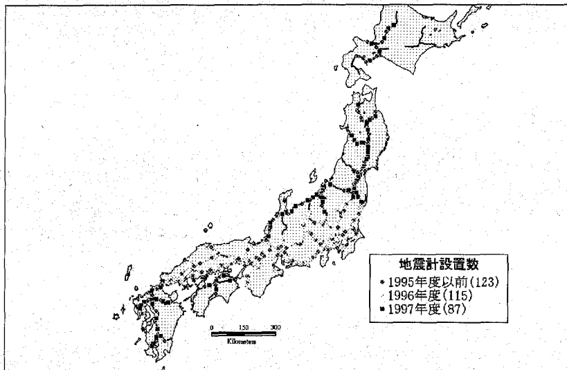
図-1 JHの地震計ネットワーク
