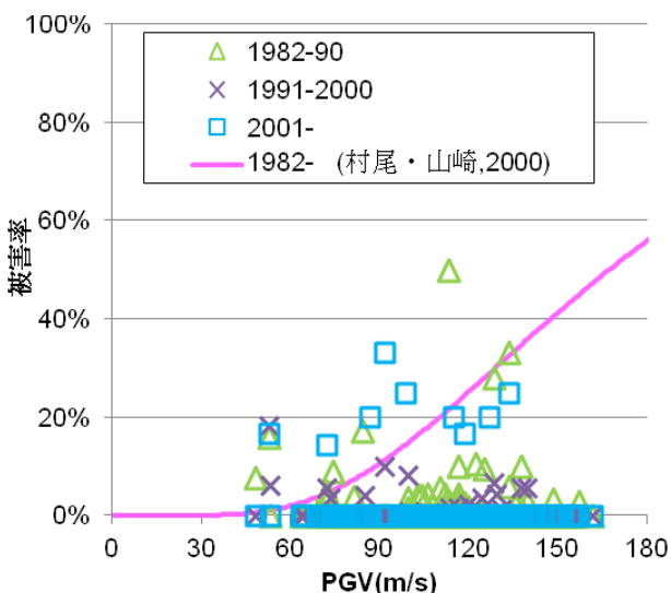
図-4 木造住宅全壊率とPGVおよび既往の被害関数との比較(1982年以降)
